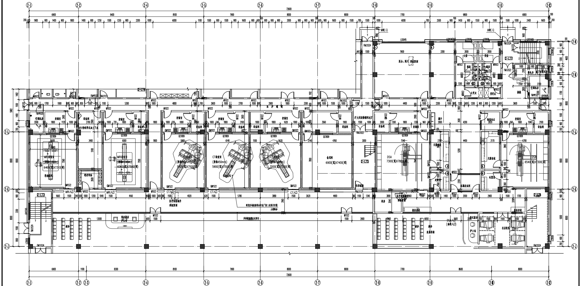
④ 外科楼一层局部平面图 1:100
